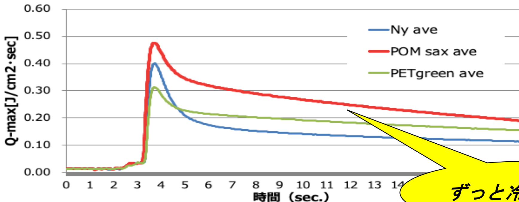
Fig.1 各種繊維の熱伝導率の経時変化
