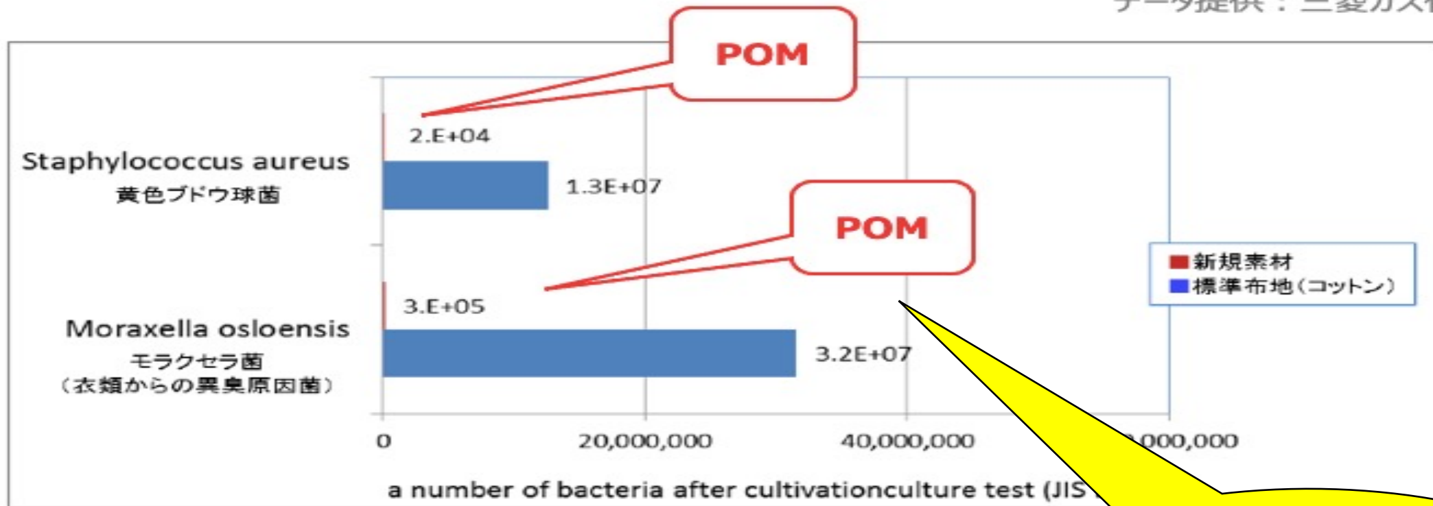
FIG.2 抗菌性試験 JIS L1902
