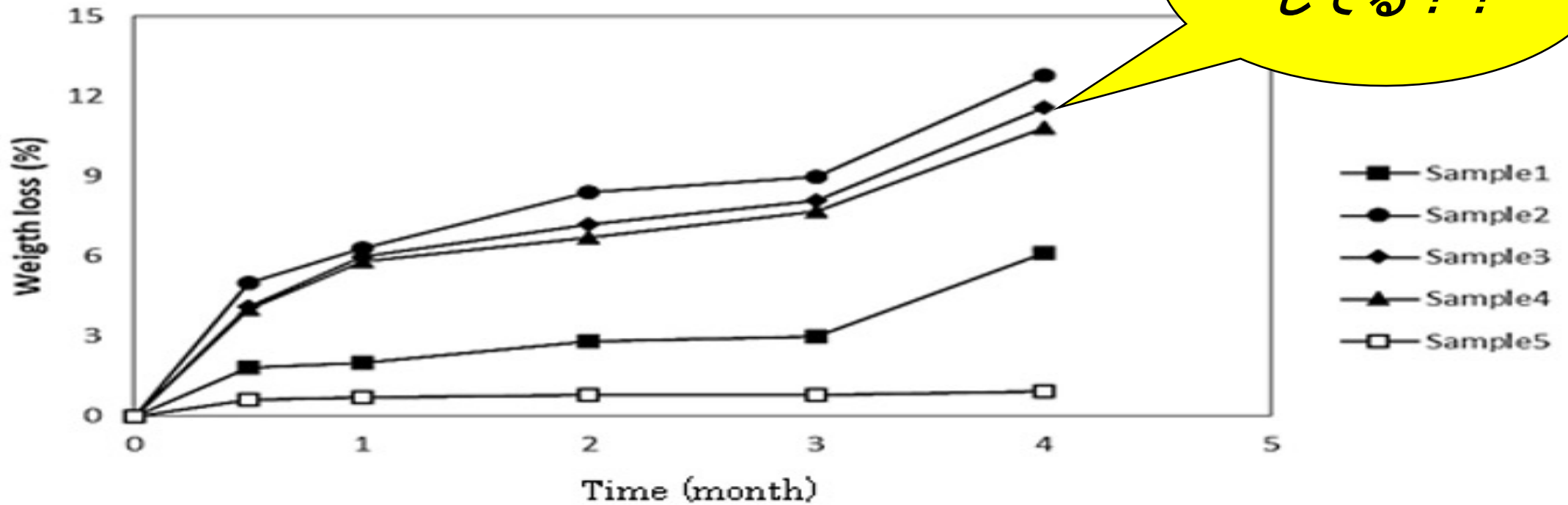
Fig-2 POM及びPOM/PLAアロイ繊維の生分解性試験
